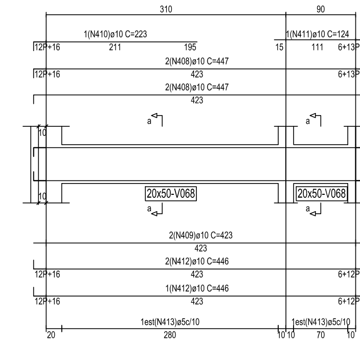
PÓRTICO: P10 COTA: 509,25 V068
