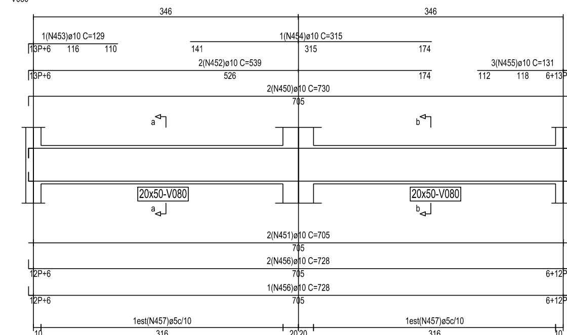
PÓRTICO: P12 COTA: 509,25 V080
