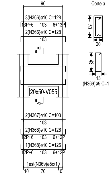
PÓRTICO: P8 COTA: 509,25 V055
