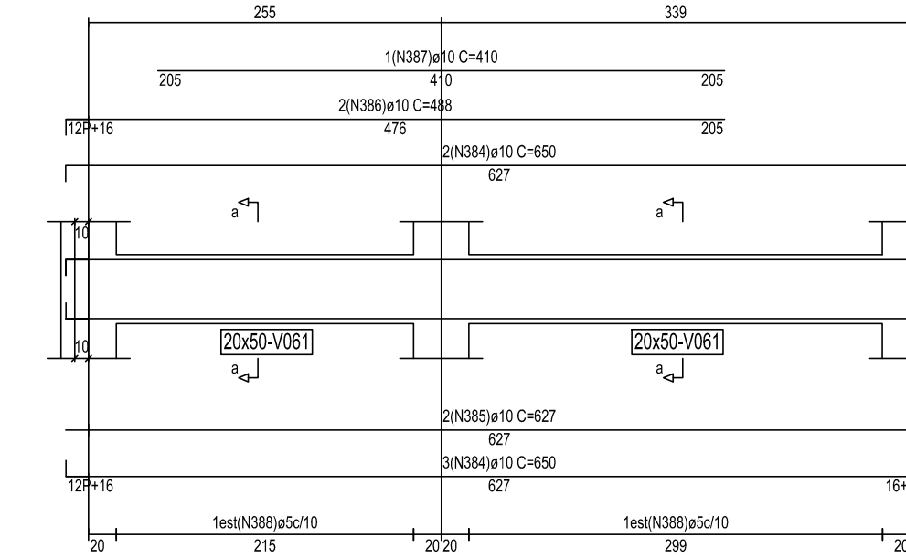
PÓRTICO: P9 COTA: 509,25 V061
