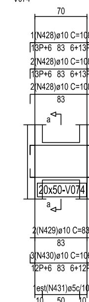
PÓRTICO: P11 COTA: 509,25 V074
