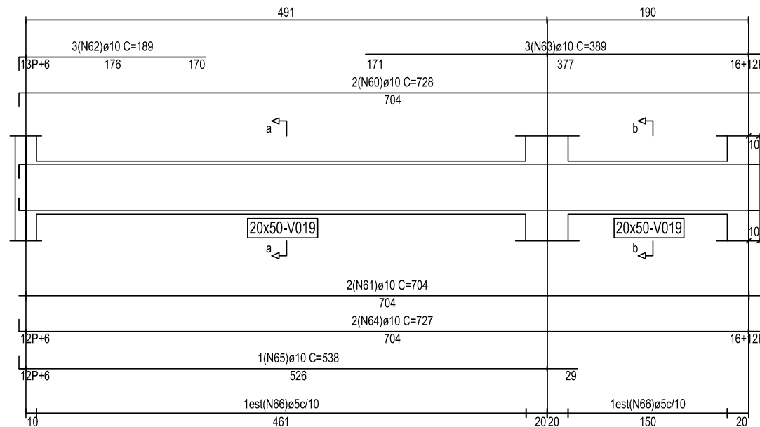
PÓRTICO: P3 COTA: 499,50 V019
