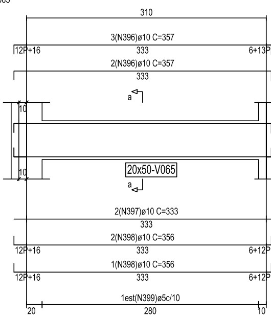
PÓRTICO: P10 COTA: 499,50 V065
