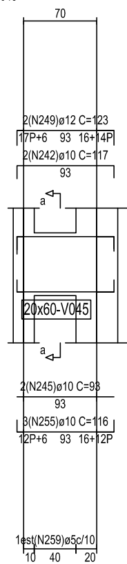
PÓRTICO: P7 COTA: 499,50 V045
