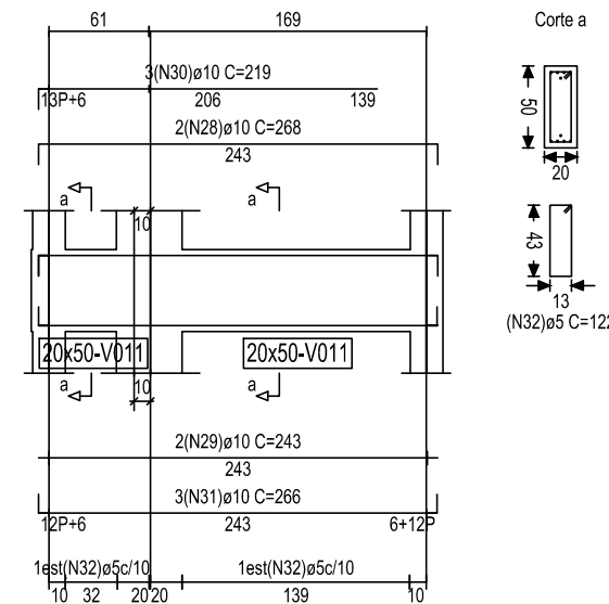
PÓRTICO: P2 COTA: 499,50 V011
